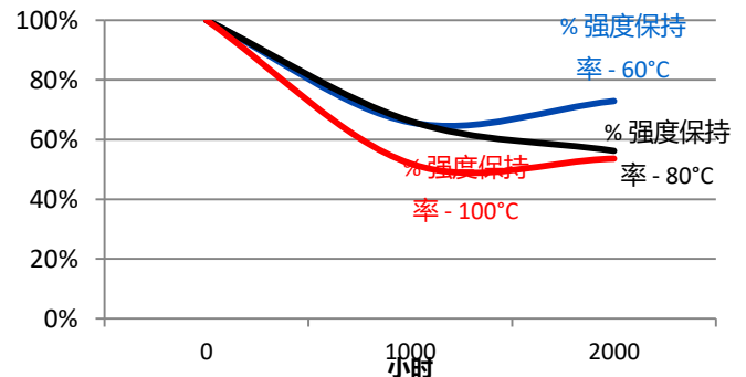
热老化曲线 (在指定温度老化, 在22°C测试)
